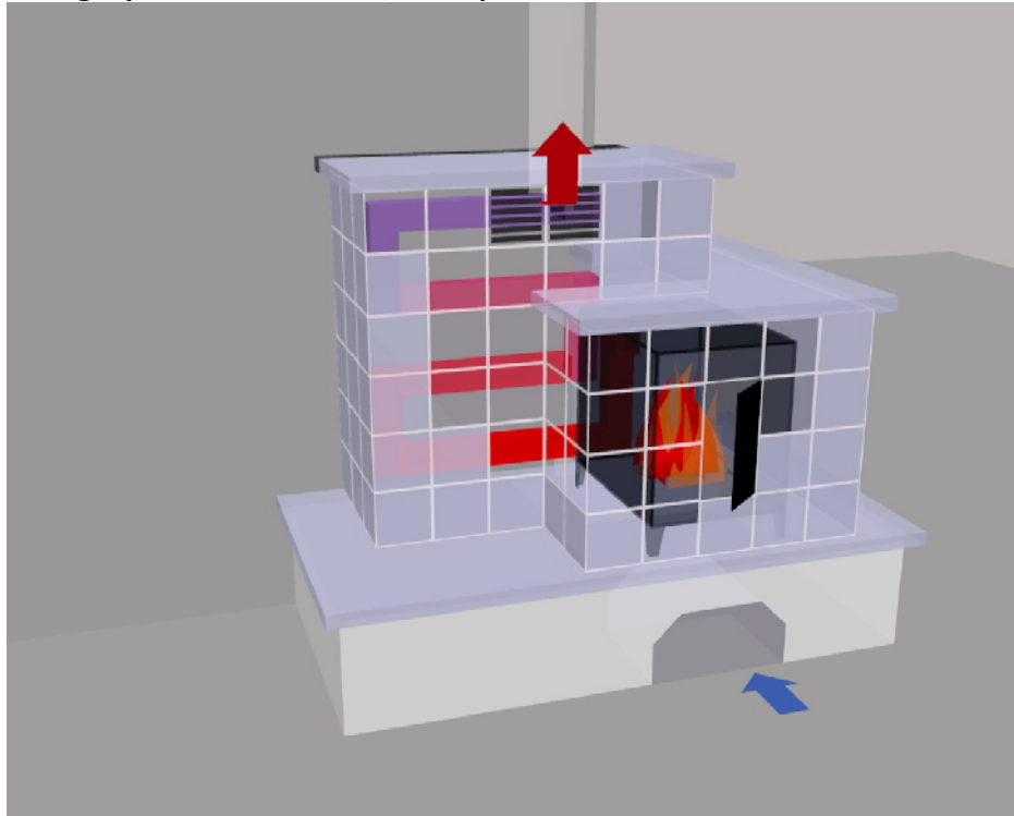
Bild 1: Technische Darstellung Kombiofen
